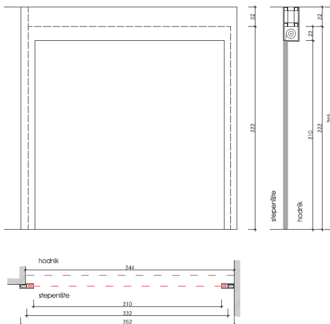
Nacrt br.6. Protupožarna zavjesa dim. 310x310 cm
