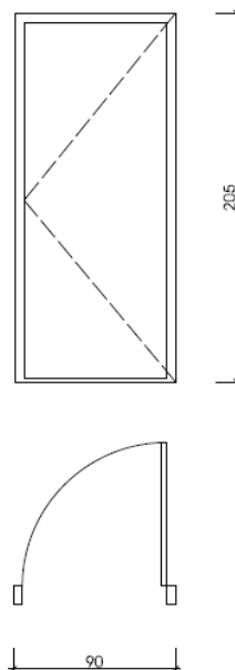
Nacrt br.8. Protupožarna vrata dim. 90x205 cm
