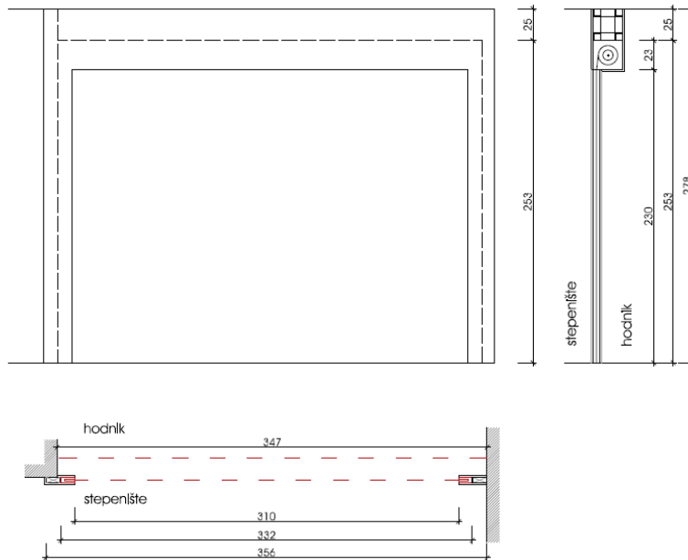
Nacrt br.7. Protupožarna zavjesa dim. 310x230 cm
