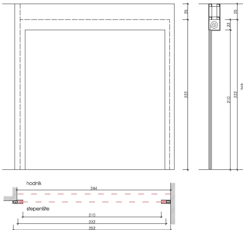
Nacrt br.4. Protupožarna zavjesa dim. 310x310 cm
