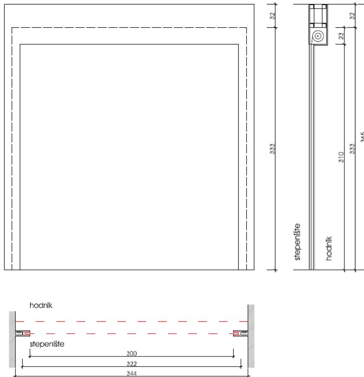
Nacrt br.5. Protupožarna zavjesa dim. 300x310 cm
