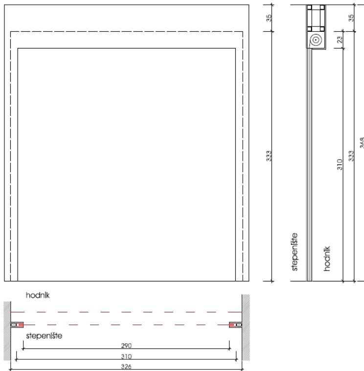
Nacrt br.1. Protupožarna zavjesa dim. 290x310 cm
