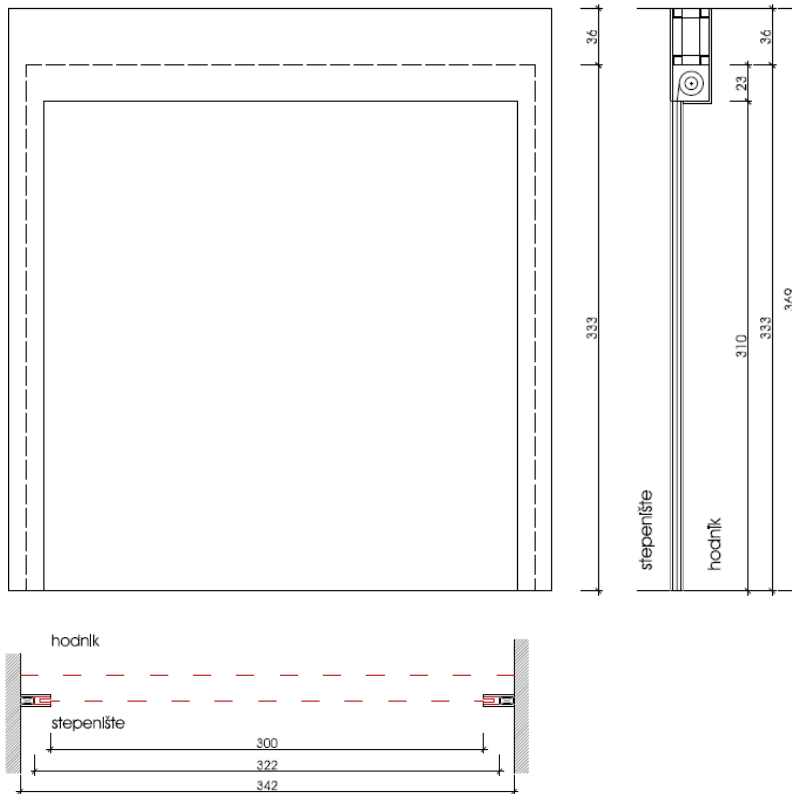
Nacrt br.3. Protupožarna zavjesa dim. 300x310 cm
