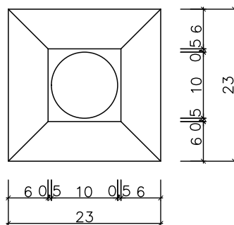
UZGLAVNI NIŠAN M 1:5
